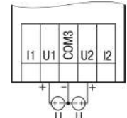
Рисунок 6 – Подключение датчиков с выходом в виде напряжения
