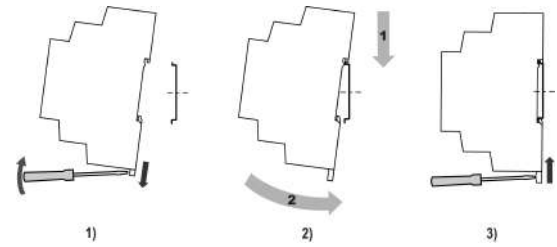
Рисунок 1 – Монтаж прибора
