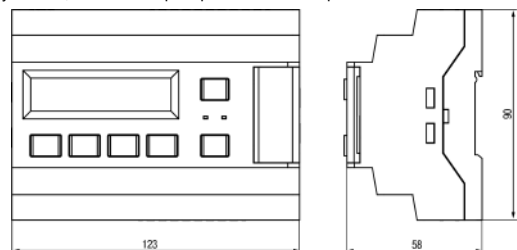
Рисунок 2 – Габаритный чертёж прибора
