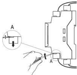
Рисунок 3 – «Быстрая» замена прибора
