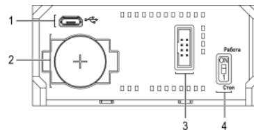
Рисунок 12 – Лицевая панель под крышкой
