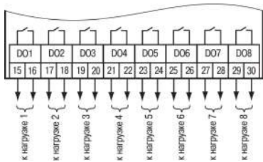
Рисунок 10 – Схема подключения нагрузки к ВЭ типа «Р»
