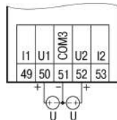
Рисунок 9 – Подключение активных датчиков с выходом типа «Напряжение 0...10 В»
