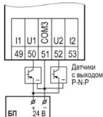
Рисунок 7 – Схема подключения к универсальным входам, работающим в дискретном режиме трехпроводных дискретных датчиков, имеющих выходной транзистор р-п-р-типа с открытым коллектором
