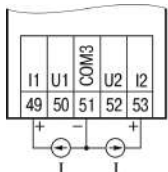
Рисунок 8 – Подключение активного датчика с выходом типа «Ток 4...20 мА»
